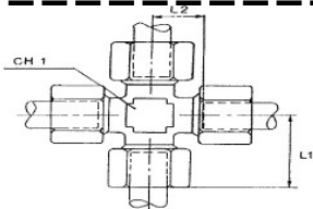
RACCORDO A CROCE SERIE S (DIN 2353)
