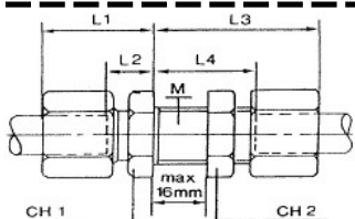
RACCORDO PASSAPARETE DIRITTO SERIE S (DIN 2353)
