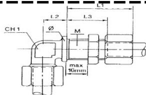
RACCORDO PASSAPARETE A GOMITO SERIE L (DIN 2353)
