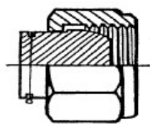
TAPPO GAS METRICO FEMMINA GIREVOLE
