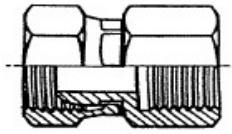
ADATTATORE FEMMINA FISSA X GAS FEMMINA GIREVOLE SEDE OGIVA
