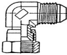
GOMITO MASCHIO JIC X FEMMINA GIR.SV.74° ELBOW JIC MALE X FEMALE SWIVEL FLARED 74°
