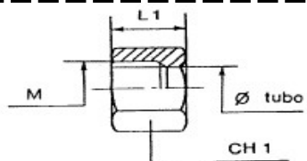
DADO DI SERRAGGIO SERIE S (DIN 2353)
