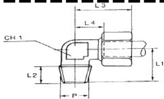
RACCORDO DI ESTREMITA' A GOMITO NPTF SERIE L (DIN 2353) EXTREMITY ELBOW FITTING NPTF SERIES L (DIN 2353)
