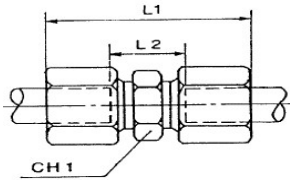
RACCORDO INTERMEDIO DIRITTO SERIE S (DIN 2353) INTERMEDIATE FITTING STRAIGHT SERIES S (DIN 2353)
