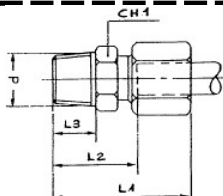
RACCORDO DI ESTREMITA' DIRITTO NPT - SERIE S (DIN 2353) EXTREMITY STRAIGHT FITTING NPT SERIES S (DIN 2353)
