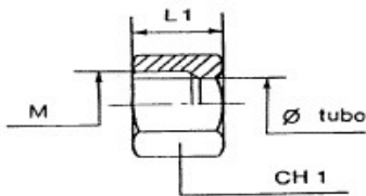
DADO DI SERRAGGIO SERIE LL (DIN 2353) LOCKING NUT SERIES LL (DIN2353)
