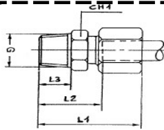
RACCORDO DI ESTREMITA' DIRITTO GAS - CONICO SERIE S (DIN 2353) EXTREMITY STRAIGHT FITTING BSP TAPERED SERIES S (DIN 2353)
