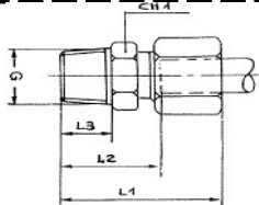
RACCORDO DI ESTREMITA' DIRITTO GAS CONICO SERIE LL (DIN 2353) EXTREMITY STRAIGHT FITTING BSP TAPERED SERIES LL (DIN 2353)
