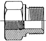
RIDUZIONE MASCHIO GAS CILINDRICO X FEMMINA FISSA GAS CILINDRICA + GUARNIZIONE REDUCTION BSP MALE X FIXED BSP FEMALE + SEAL
