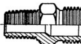
NIPPLIO RIDOTTO GAS CILINDRICO SVASATO X GAS CILINDRICO SVASATO METRICO REDUCED NIPPLE BSP FLARED X BSP FLARED METRIC
