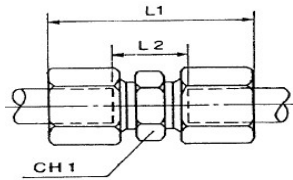
RACCORDO INTERMEDIO DIRITTO SERIE L (DIN 2353) INTERMEDIATE FITTING STRAIGHT SERIES L (DIN 2353)
