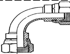
ADATTATORE 90° GAS FEMMINA GIREV. SEDE OGIVA X GAS FEMMINA GIREV. SEDE OGIVA
