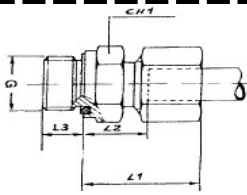
RACCORDO DI ESTREMITA' DIRITTO GAS CILINDRICO CON GUARNIZIONE PIANA SERIE S (DIN 2353) EXTREMITY STRAIGHT FITTING BSP WITH GASKET FLAT SERIES S (DIN 2353)
