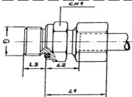
RACCORDO DI ESTREMITA' DIRITTO GAS CILINDRICO CON GUARNIZIONE PIANA SERIE L (DIN 2353) EXTREMITY STRAIGHT FITTING BSP WITH GASKET FLAT SERIES L (DIN 2353)
