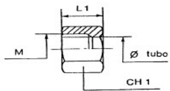
DADO DI SERRAGGIO SERIE L (DIN 2353)
