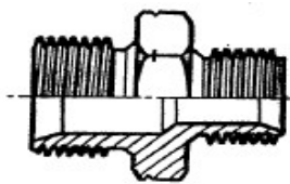
NIPPLIO RIDOTTO GAS CILINDRICO SVASATO X GAS CILINDRICO SVASATO METRICO REDUCED NIPPLE BSP FLARED X BSP FLARED METRIC
