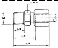
RACCORDO DI ESTREMITA' DIRITTO GAS - CONICO SERIE L (DIN 2353) EXTREMITY STRAIGHT FITTING BSP TAPERED SERIES L (DIN 2353)
