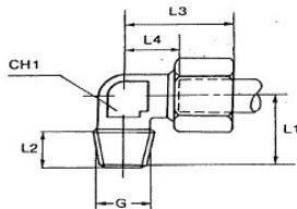
RACCORDO DI ESTREMITA' A GOMITO GAS - CONICO SERIE S (DIN 2353) EXTREMITY ELBOW FITTING BSP TAPERED SERIES S (DIN 2353)
