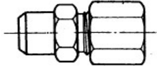
ESTREMITA' A SALDARE DIN 2353 SERIE S EXTREMITY TO BE WELDED DIN 2353 SERES S
