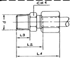
RACCORDO DI ESTREMITA' DIRITTO NPT - SERIE L (DIN 2353) EXTREMITY STRAIGHT FITTING NPT SERIES L (DIN 2353)
