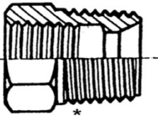
RIDUZIONE MASCHIO GAS CONICO X FEMMINA FISSA GAS CILINDRICA REDUCTION BSPT MALE X FIXED BSP FEMALE
