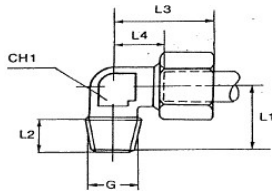
RACCORDO DI ESTREMITA' A GOMITO GAS - CONICO SERIE L (DIN 2353) EXTREMITY ELBOW FITTING BSP TAPERED SERIES L (DIN 2353)
