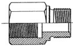
RIDUZIONE MASCHIO GAS CILINDRICO X FEMMINA FISSA GAS CILINDRICA + GUARNIZIONE REDUCTION BSP MALE X FIXED BSP FEMALE + SEAL
