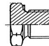
TAPPO GAS CILINDRICO PIANO METRICO MASCHIO
