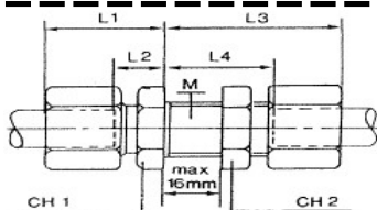
RACCORDO PASSAPARETE DIRITTO SERIE L (DIN 2353)
