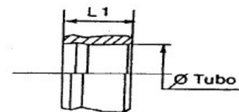
ANELLO TAGLIENTE SERIE S (DIN 2353)
