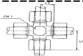
RACCORDO A CROCE SERIE L (DIN 2353)
