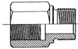
RIDUZIONE MASCHIO GAS CILINDRICO X FEMMINA FISSA GAS CILINDRICA CON GUARNIZIONE REDUCTION BSP MALE X FIXED BSP FEMALE + SEAL
