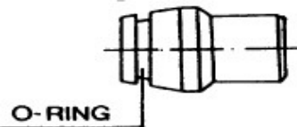
TAPPO DIN 2353 CON OR TOP DIN 2353 WITH OR
