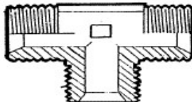
TEE MASCHIO-MASCHIO-MASCHIO GAS CILINDRICO TEE MALE-MALE-MALE BSP
